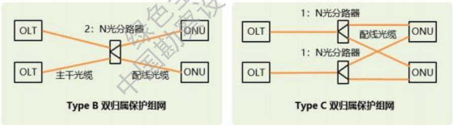
图表 2-20 F5G 全光网 Type B 和 Type C 双归属保护
