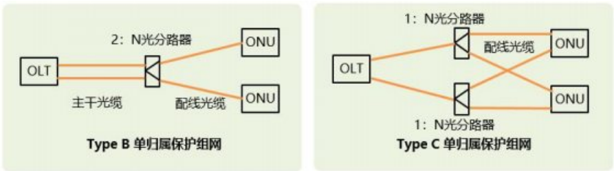
图表 2-21 F5G 全光网 Type B 和 Type C 单归属保护
