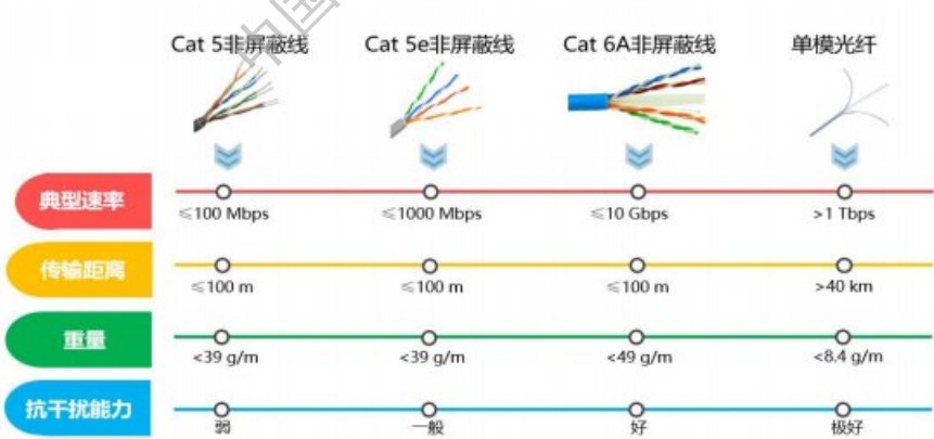
图表 2-14 网线和光纤的传输性能/重量对比
